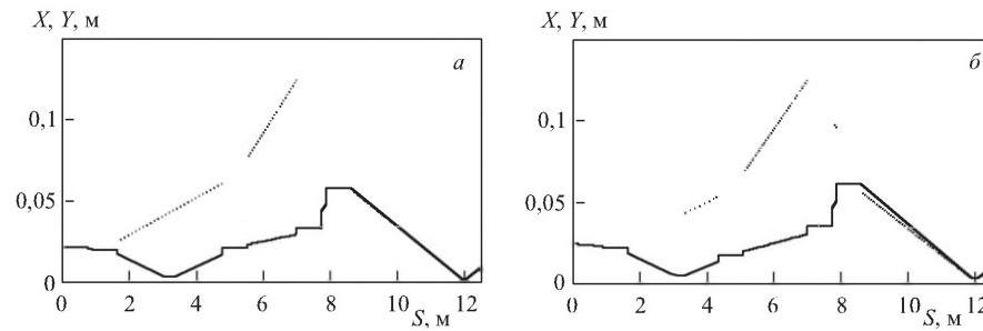
Рис. 3. Огибающие пучка X, Y вдоль канала для значений эмиттаиса 25 \pi мм · мрад (a) и 50 \pi мм · мрад (б). Пунктиром показана огибающая Y
