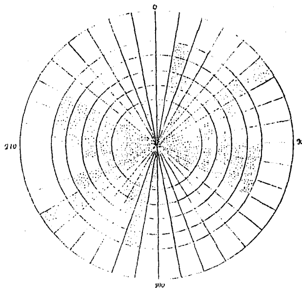
Figura N° 3. Diagrama de juntas riolitas de Cretácico Inferior. Cerro Arequita, departamento de Lavalleja.
