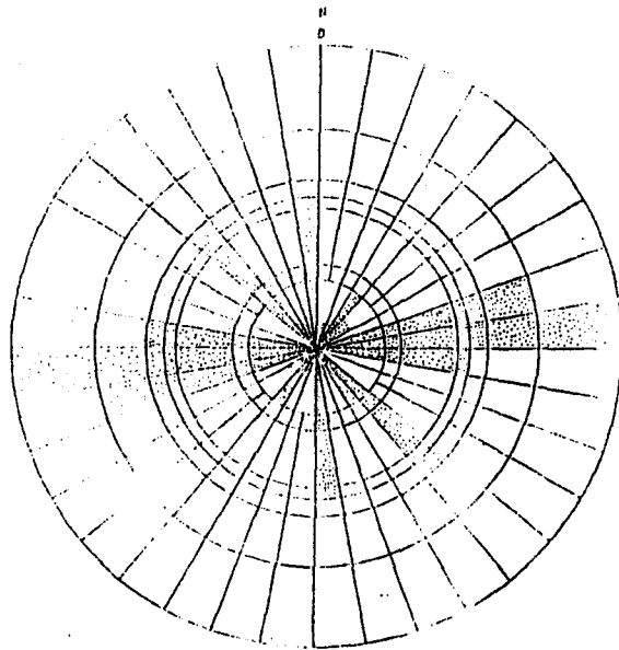
Figura N° 2. Diagrama de juntas Formación Arapey, Ruta 26, km. 199-191.
