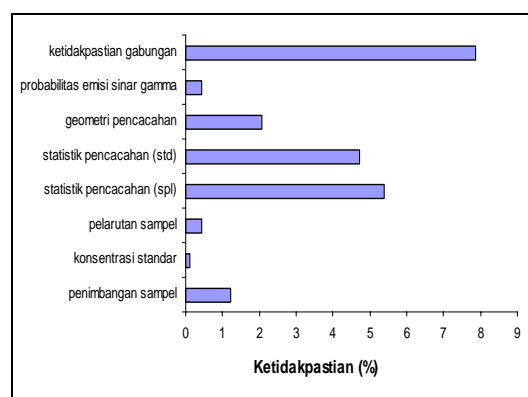
Gambar 2. Ketidakpastian relatif masing-masing komponen dan ketidakpastian gabungan
