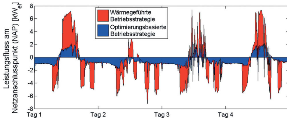
Abbildung 5 Wärmespeicher steigern Netzdienstlichkeit von PV-Wärmepumpensystemen: Blau = Betriebsweise mit Speicher Rot = Betriebsweise ohne Speicher (Fraunhofer IWES)
