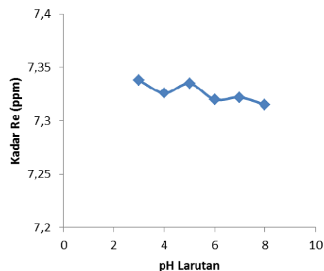
Gambar 5. Pengaruh pH larutan terhadap kadar Re dalam fasa organik.
