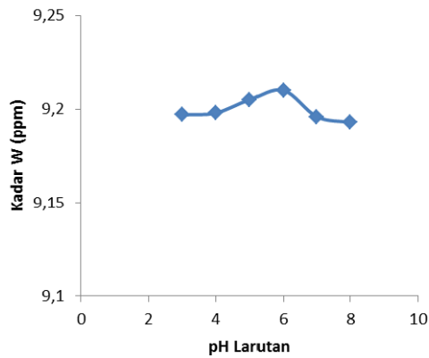
Gambar 6. Pengaruh pH larutan terhadap kadar W dalam fasa air.
