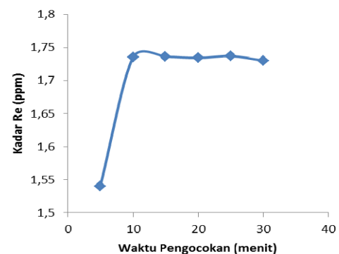
Gambar 1. Pengaruh waktu pengocokan terhadap kadar Re dalam fase organik.
