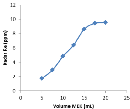
Gambar 3. Pengaruh volume pelarut MEK terhadap kadar Re dalam fase organik.
