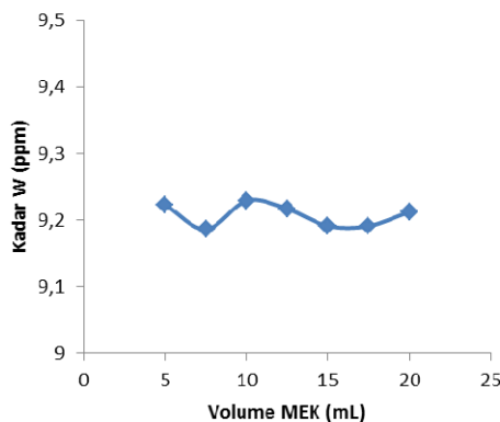
Gambar 4. Pengaruh volume pelarut MEK terhadap kadar W dalam fase air.
