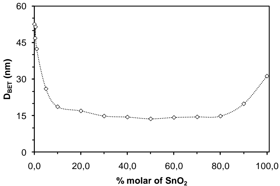
Figura 5: Tamanho de partícula calculado a partir da área de superfície específica e da densidade em função da concentração de SnO 2 .
