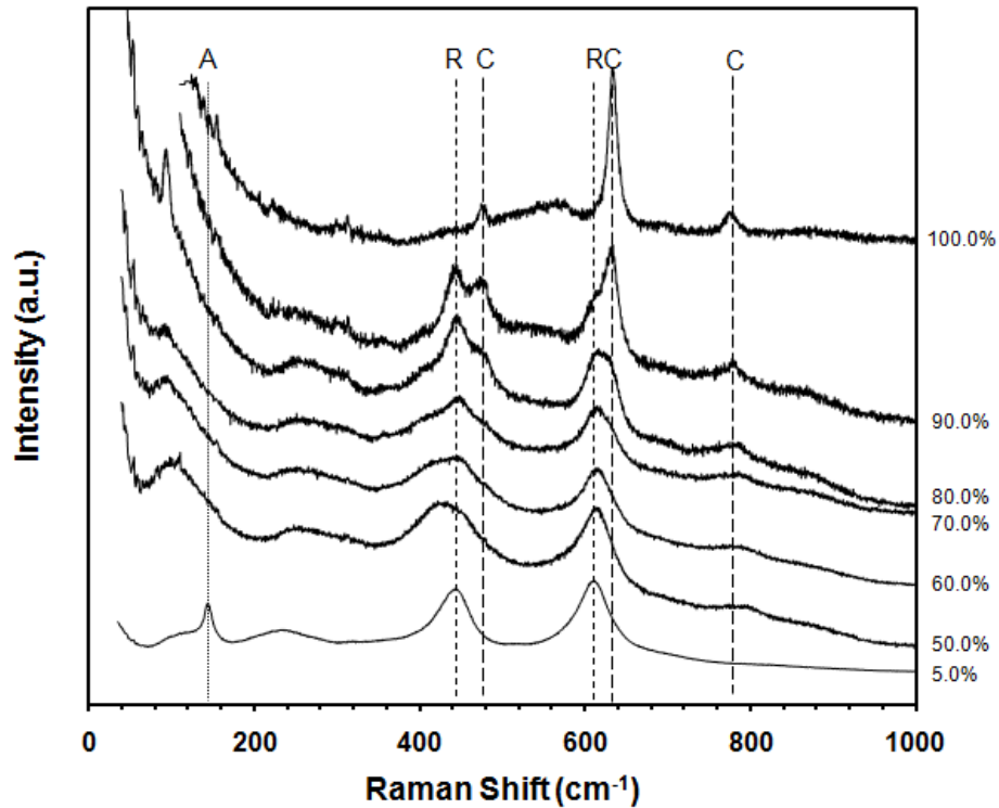
Figura 2: Espectros Raman dos pós com concentrações de 50,0 à 100,0% de SnO 2 .
