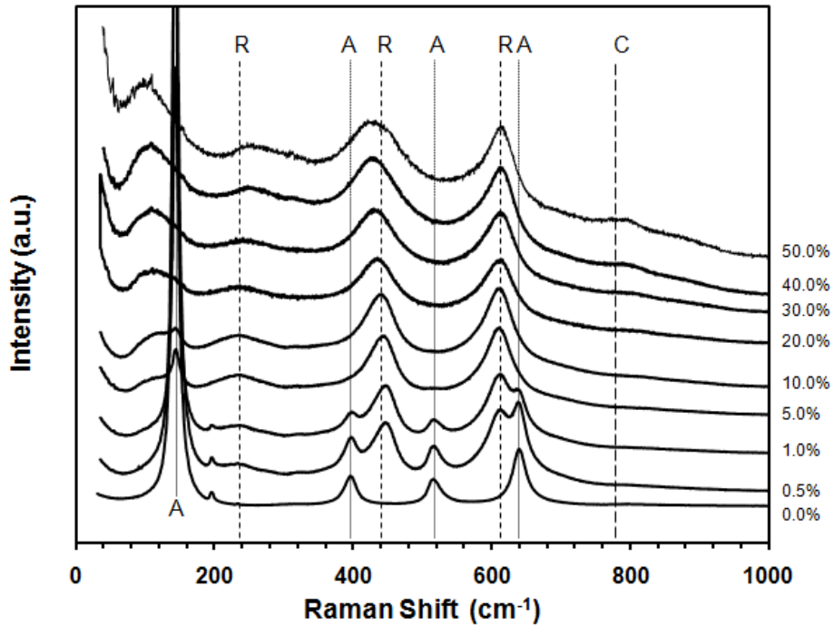
Figura 1: Espectros Raman dos pós com concentrações de 0,0 à 50,0% em mol de \text{SnO}_2 .
