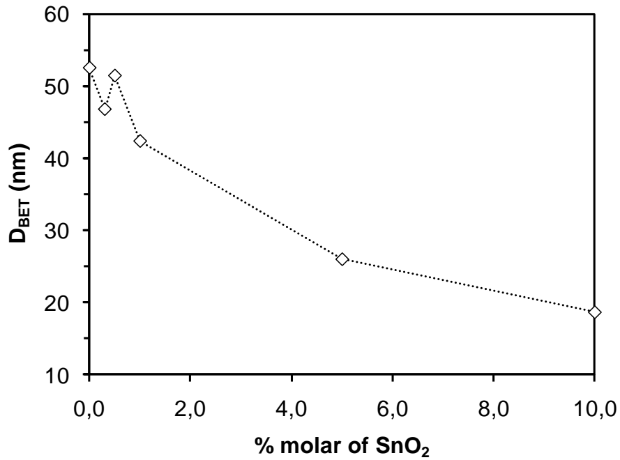
Figura 4: Tamanho de partícula calculado a partir da área de superfície específica e da densidade em função da concentração de SnO 2 de pós contendo até 10,0% molar.
