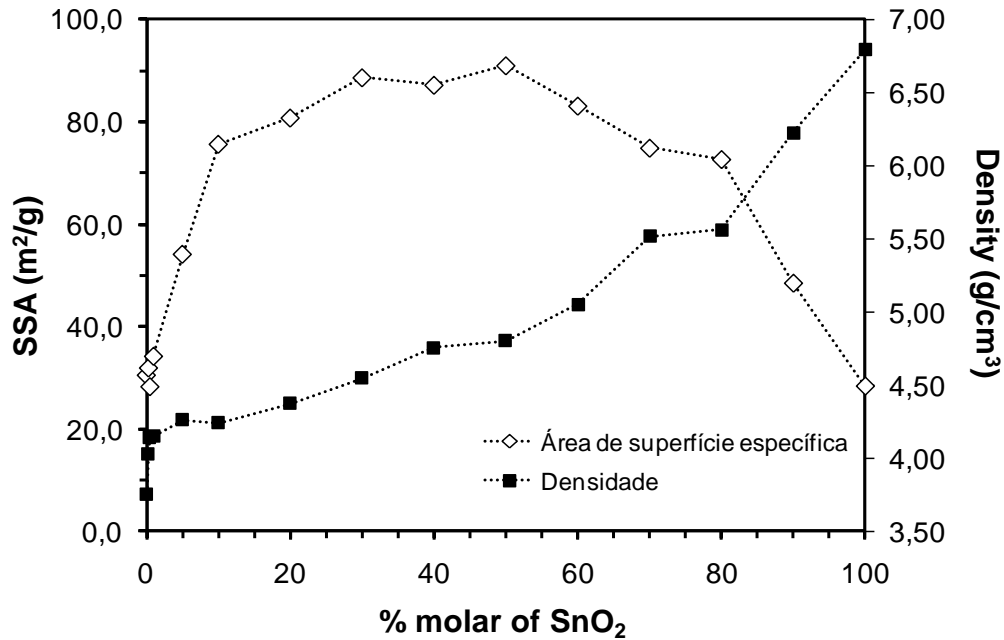
Figura 3: Área de superfície específica e densidade em função da concentração de SnO 2 .
